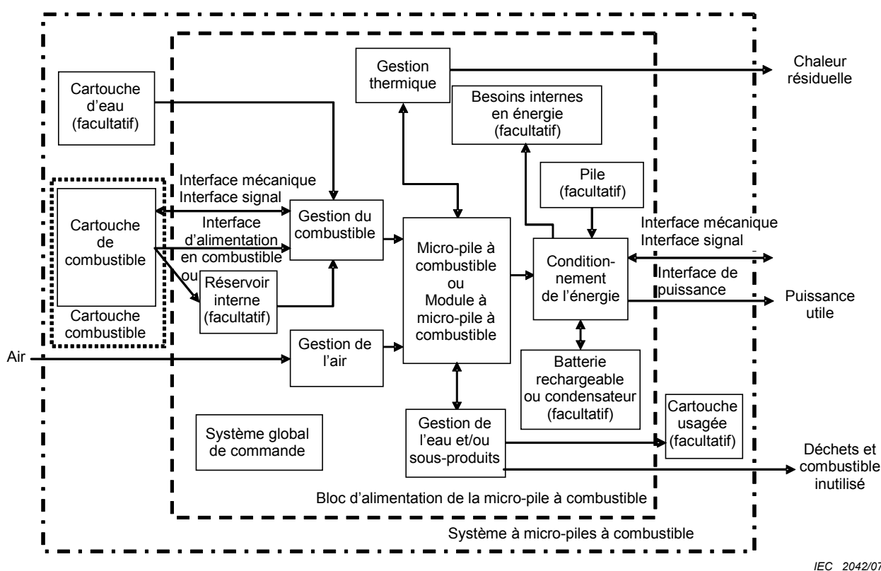
Figure 1 – Dispositif fonctionnel abordé dans le domaine d'application de cette norme
